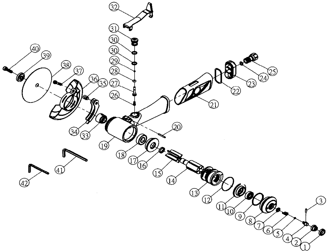
PT-387 カットオフツール 部品図
