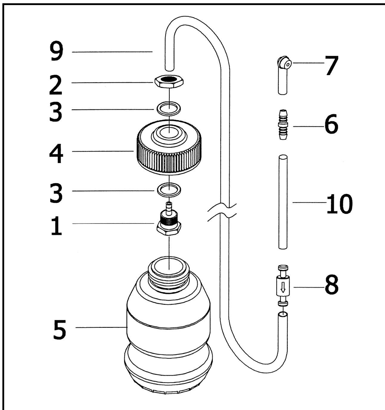
QS-2121 ブレーキフリードキャッチタンク 部品図
