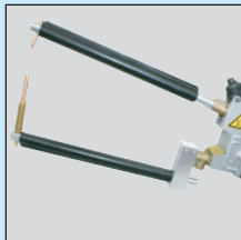
ワイドアダプターセット付ロングアーム (MDL+MDWS SET) 左: チップアダプター TTA-70 右: ワイドアダプター MDWS
