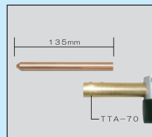
左: タイヤハウス用送り側チップ (ST135-12) 右: チップアダプター (TTA-70)
