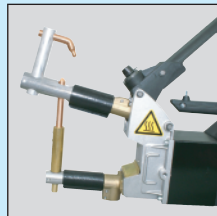
タイヤハウスアーム (MDT)
