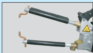
ミディアムアーム300mm (MDM)
