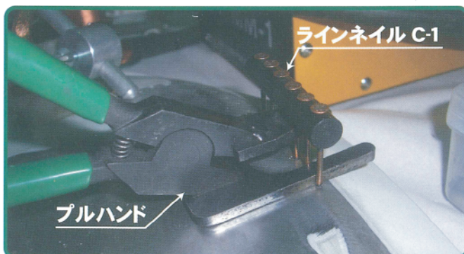
ラインネイルをプルハンドを使って
