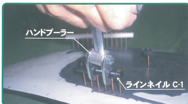
ハンドプーラーを使ってハンマリング
