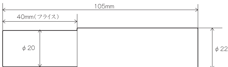
VG-105 (材質アルミ)
