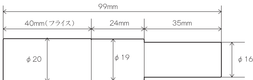
YA-99 (材質真鍮)
