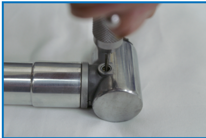
② タップでオイルプラグの穴にネジ込みます。
